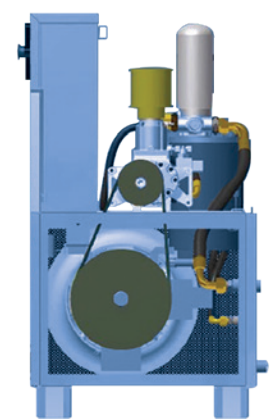
Automatisches Riemenspannsystem
